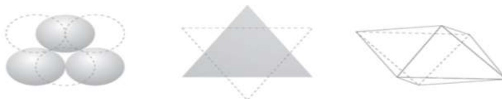
Figura 6. Apilamiento de capas compactadas formación de octaedros. (Guía interactiva de minerales y rocas. Universidad Politécnica de Madrid).
