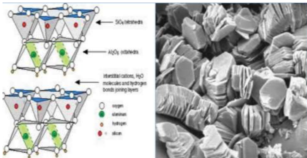
Figura 8. Diagrama esquemático y de foto microscopía electrónica de la caolinita (Fuente: Alvarado, A., Mata, R & Chinchilla, M., 2014).
