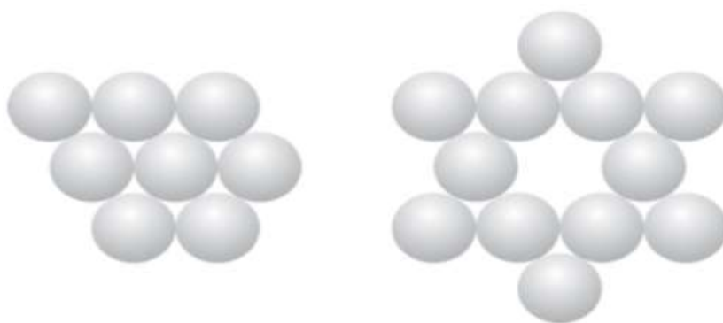
Figura 5. Capa compacta y no compacta (hexagonal) de la estructura de los filosilicatos. (Guía interactiva de minerales y rocas. Universidad Politécnica de Madrid).
