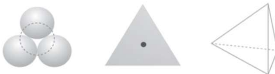
Figura 7. Apilamiento de una capa compactada y una no compactada, formación de tetraedros. (Guía interactiva de minerales y rocas. Universidad Politécnica de Madrid).
